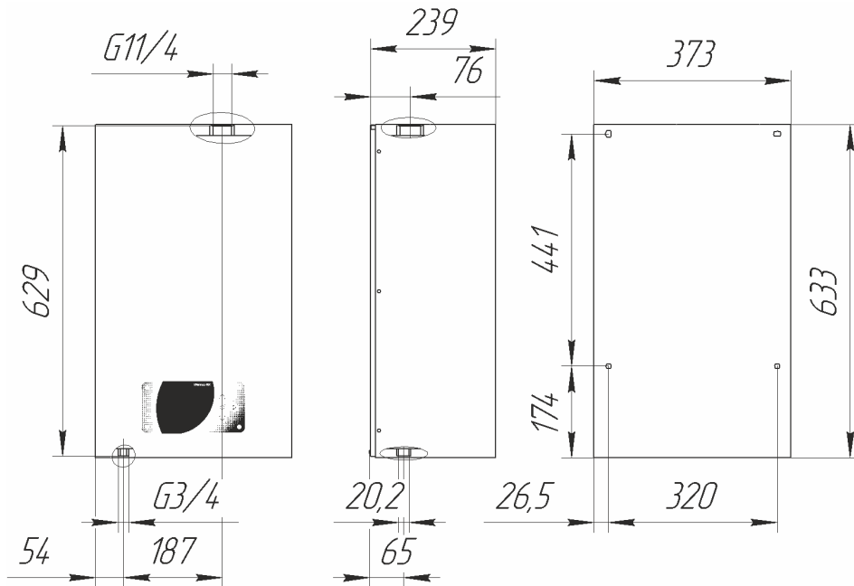
Рисунок 4. Габаритные и присоединительные размеры
