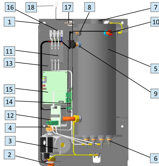
Рисунок 2. Внешний вид прибора со снятым кожухом
