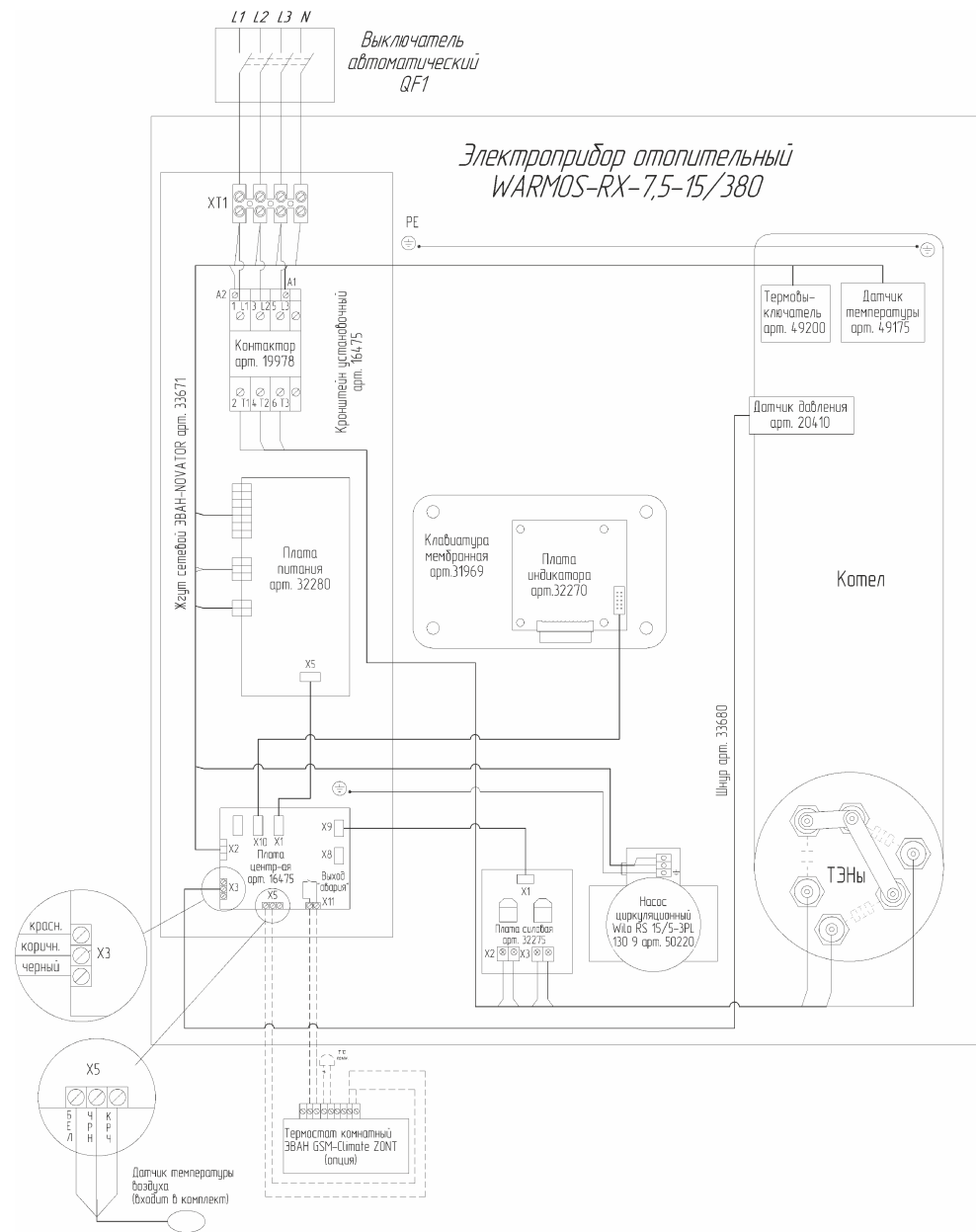
Рисунок 8 Схема подключения WARMOS-RX -7,5-15 (380)
