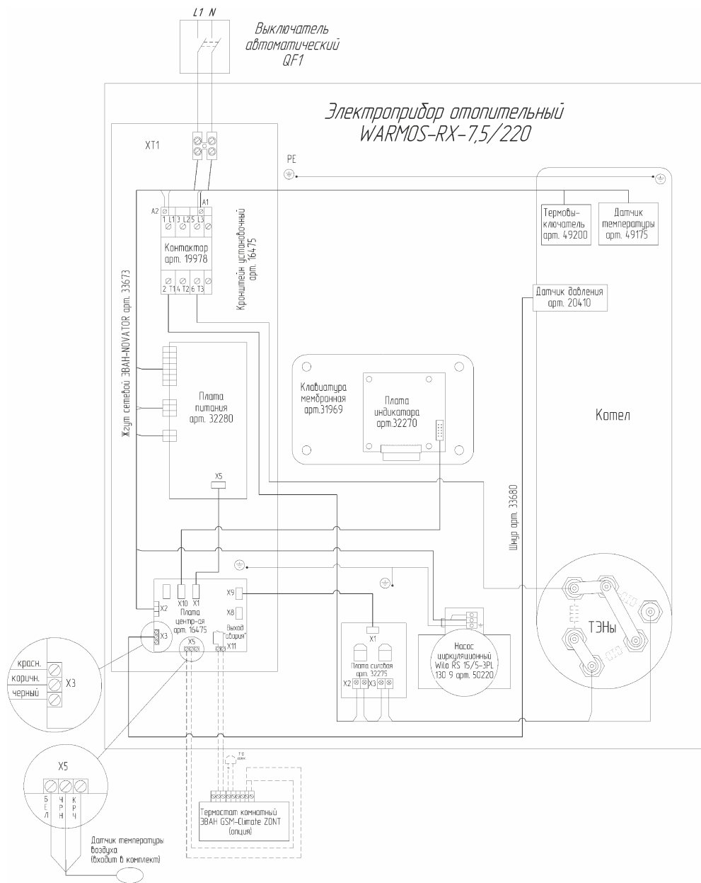
Рисунок 7 Схема подключения WARMOS-RX -7,5 (220 В)
