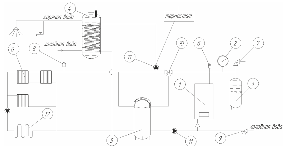
Рисунок 5. Возможная схема системы отопления и ГВС.
