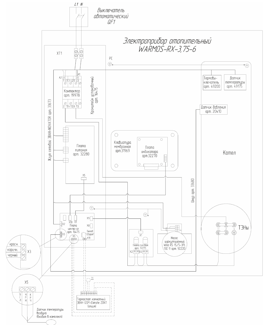
Рисунок 6 Схема подключения WARMOS-RX -3.75-6
