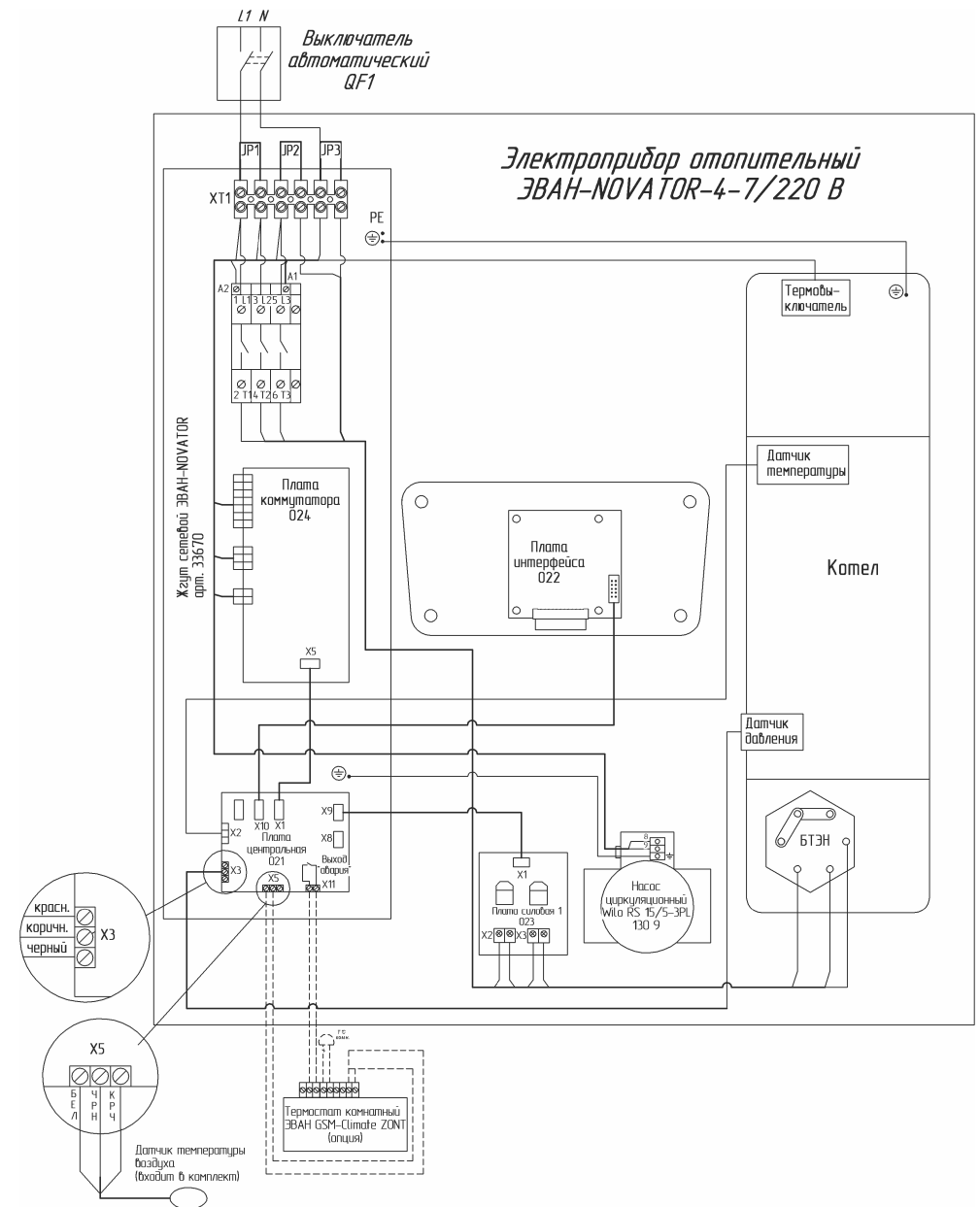
Рисунок 6 Схема подключения ЭВАН NOVATOR -4-7/ 220 В
