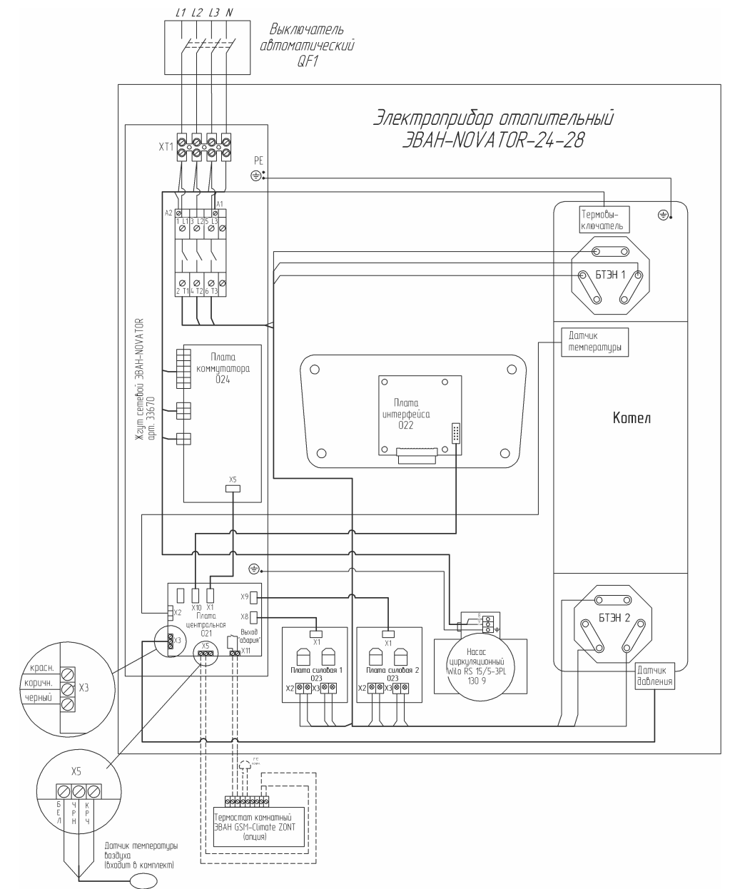
Рисунок 10 Схема подключения ЭВАН NOVATOR -24, -28
